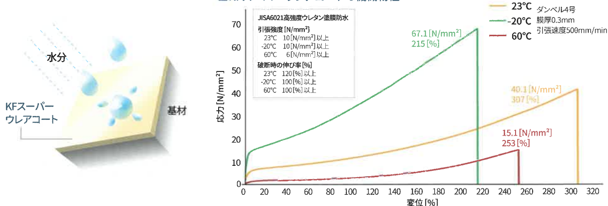
■KFスーパーウレアコートの機械物性
